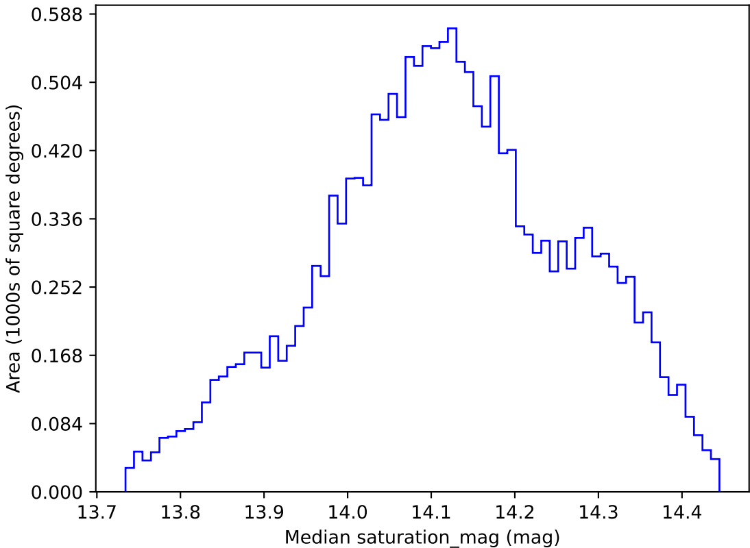
weather_cloudso4v3.4_10yrs WFD z band: Median saturation_mag
