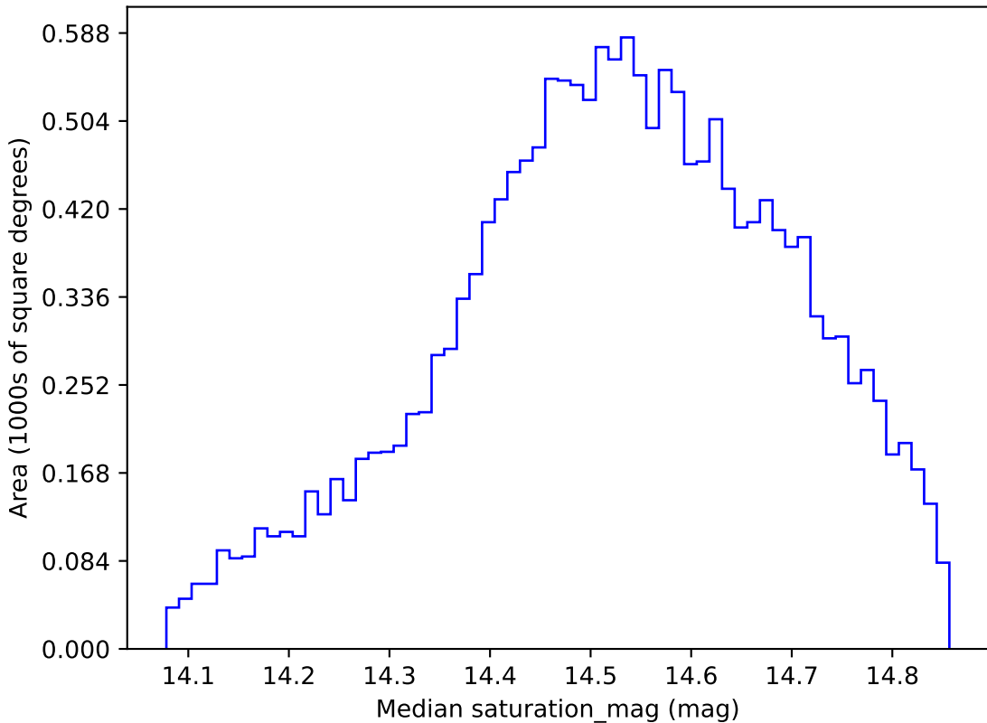
weather_cloudso4v3.4_10yrs WFD i band: Median saturation_mag
