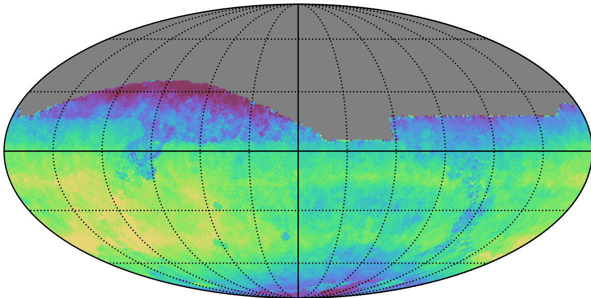
weather_cloudso4v3.4_10yrs All sky i band: Median saturation_mag
