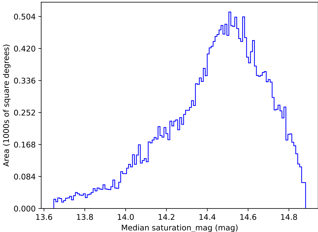
weather_cloudso4v3.4_10yrs All sky i band: Median saturation_mag
