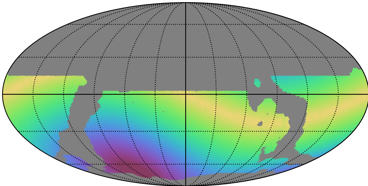
weather_cloudso4v3.4_10yrs WFD y band: Max solarElong
