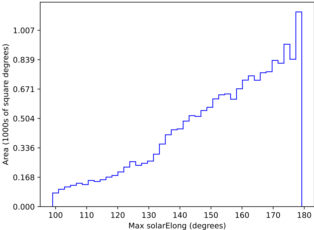
weather_cloudso4v3.4_10yrs WFD y band: Max solarElong
