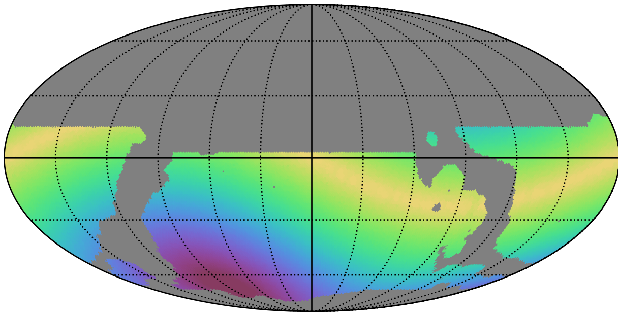
weather_cloudso4v3.4_10yrs WFD i band: Max solarElong
