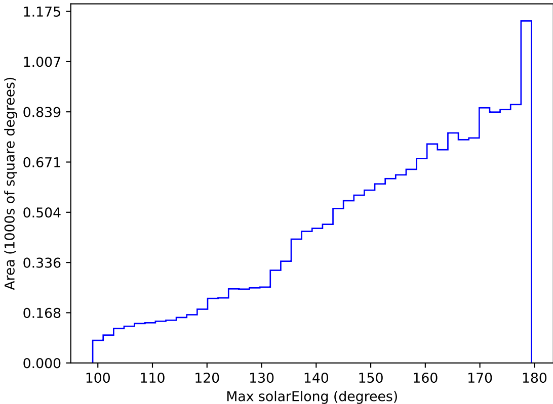
weather_cloudso4v3.4_10yrs WFD i band: Max solarElong
