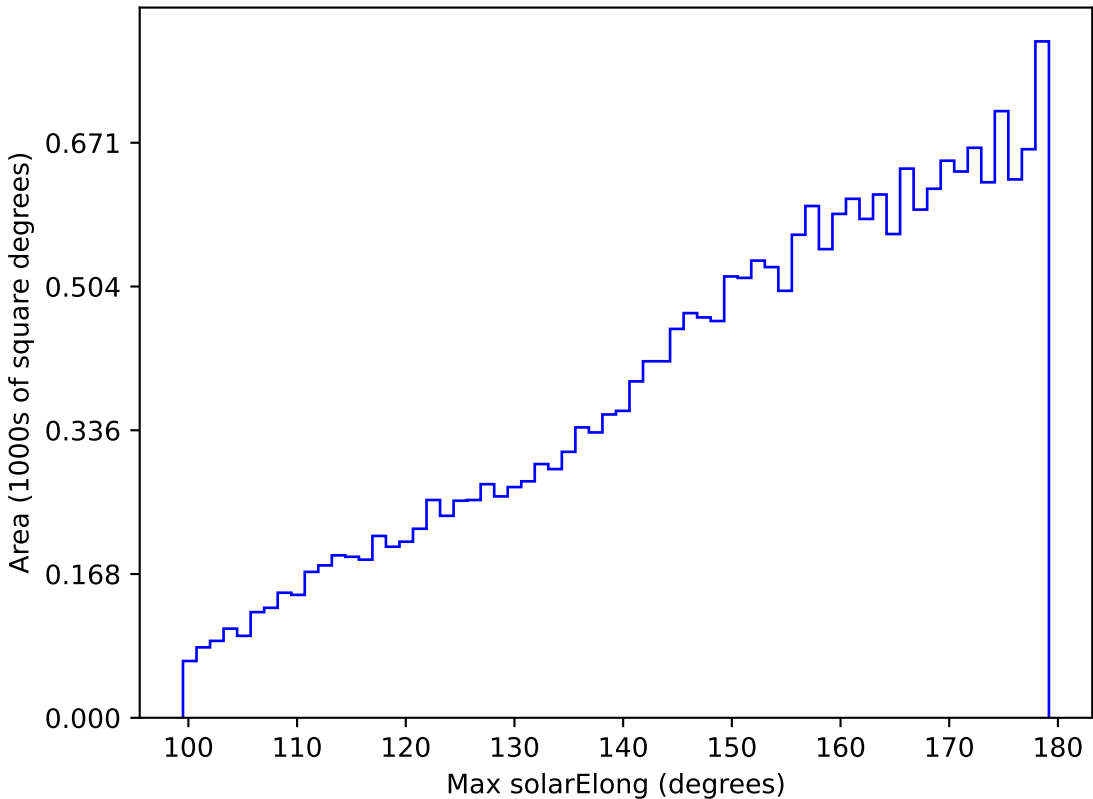
weather_cloudso4v3.4_10yrs All sky y band: Max solarElong
