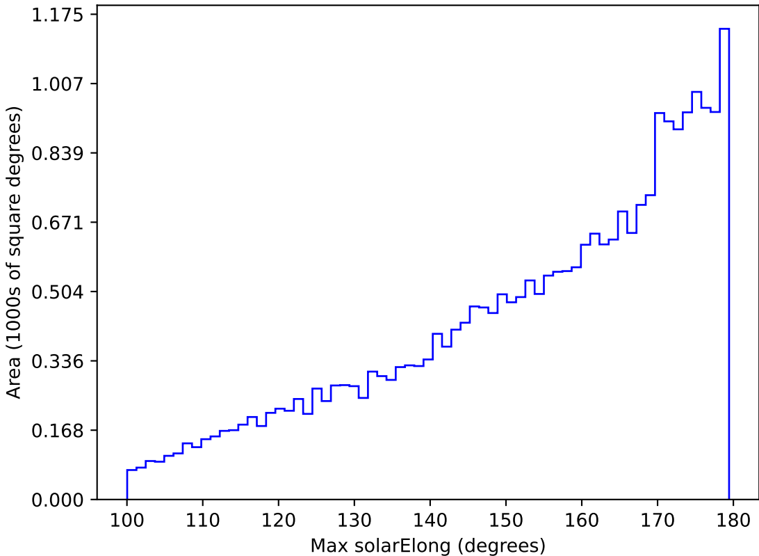
weather_cloudso4v3.4_10yrs All sky i band: Max solarElong
