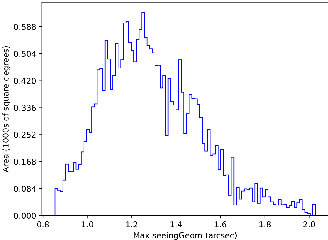
weather_cloudso4v3.4_10yrs Yr 1 y band: Max seeingGeom
