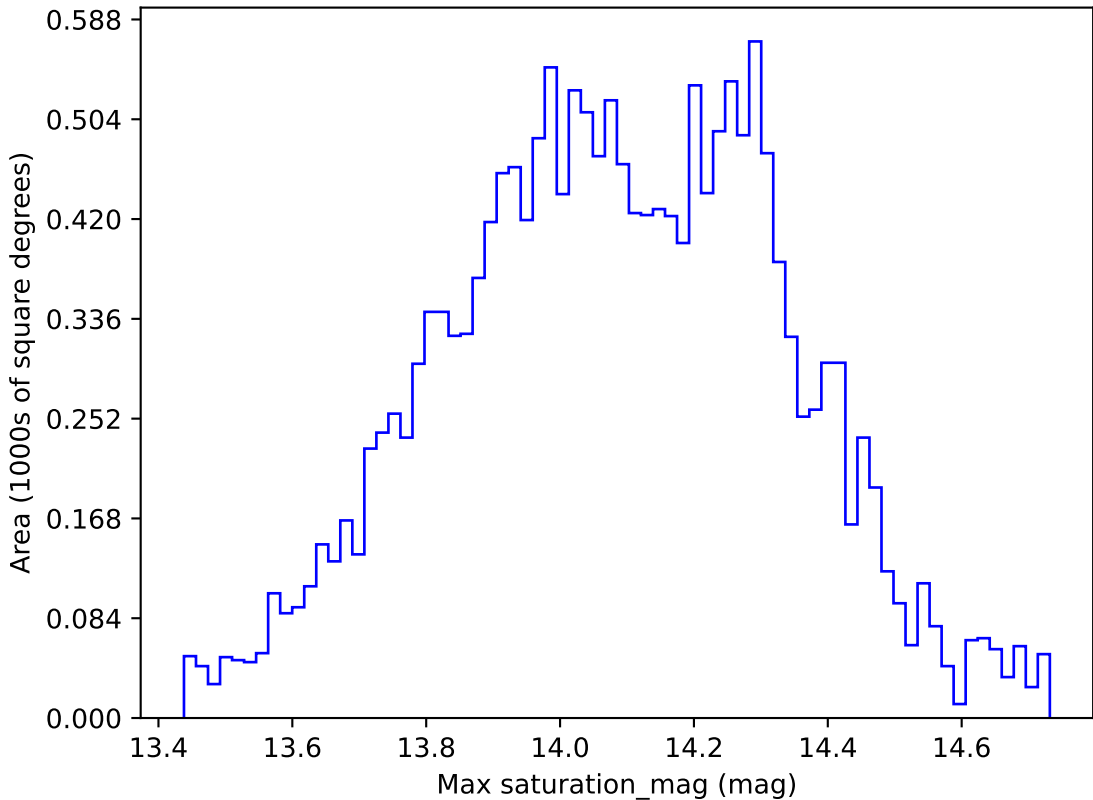
weather_cloudso4v3.4_10yrs WFD u band: Max saturation_mag
