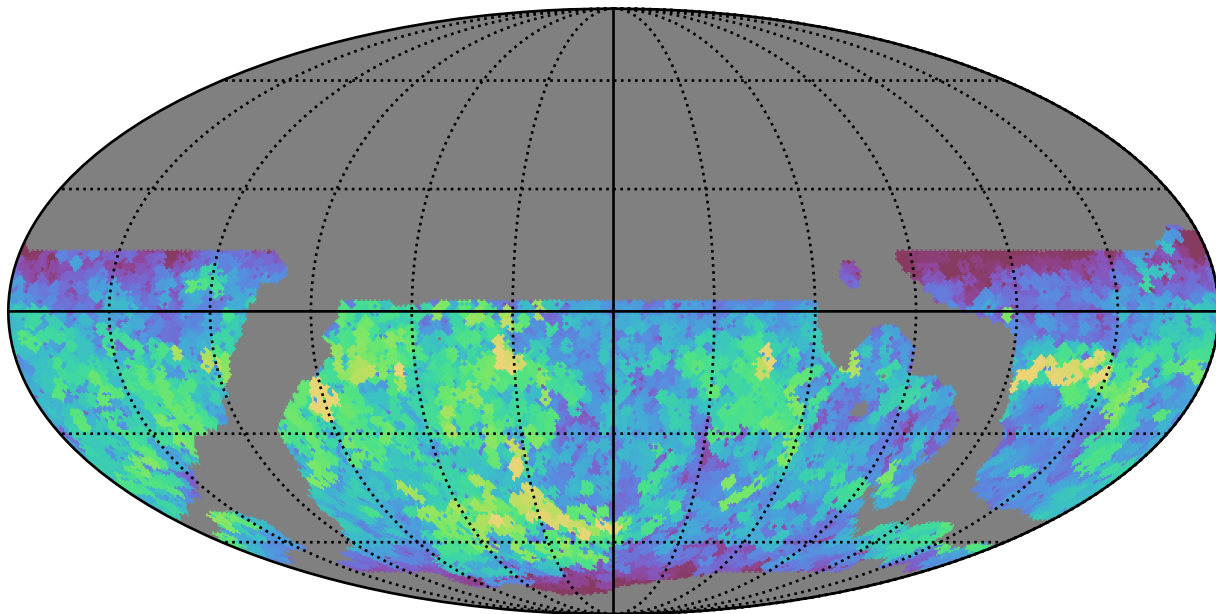
weather_cloudso4v3.4_10yrs WFD r band: Max saturation_mag
