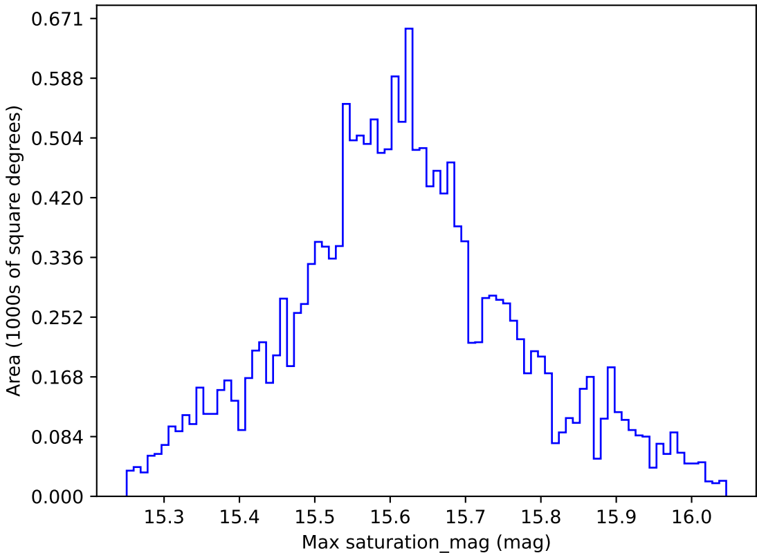
weather_cloudso4v3.4_10yrs WFD i band: Max saturation_mag
