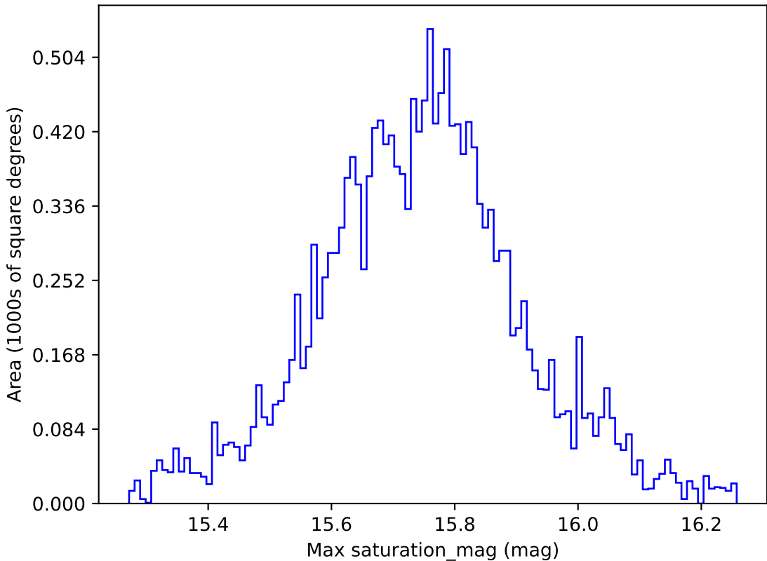
weather_cloudso4v3.4_10yrs WFD g band: Max saturation_mag
