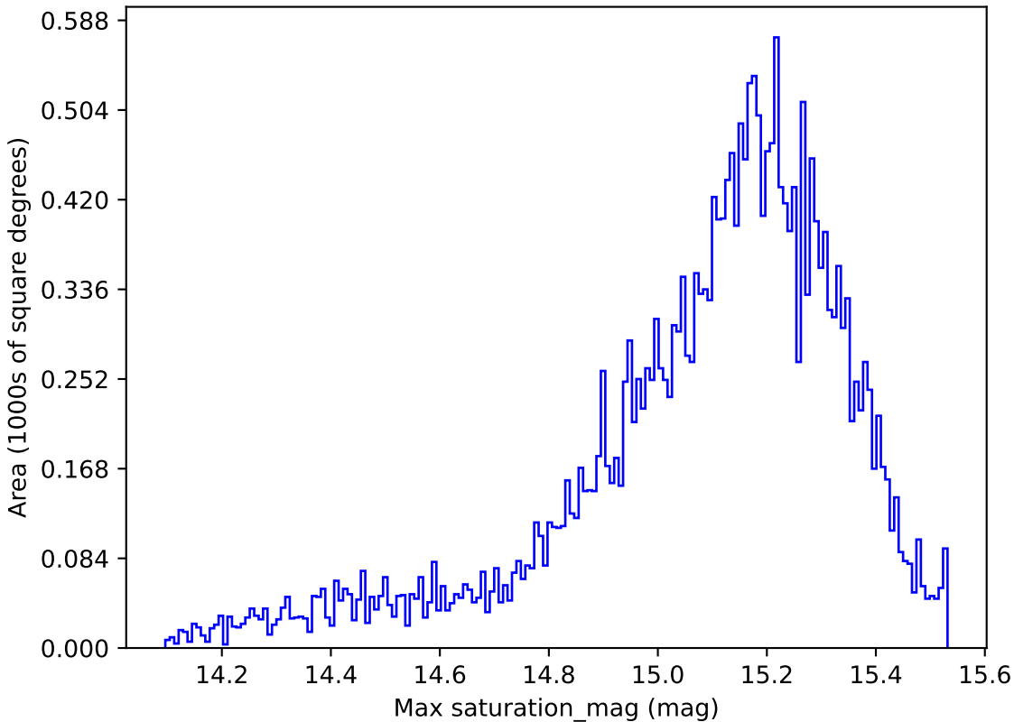
weather_cloudso4v3.4_10yrs All sky z band: Max saturation_mag
