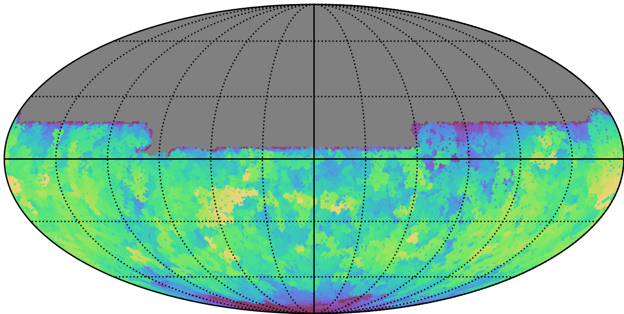
weather_cloudso4v3.4_10yrs All sky u band: Max saturation_mag
