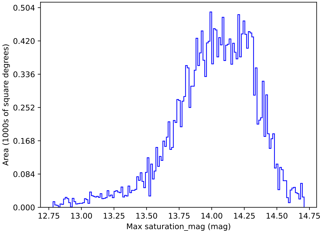
weather_cloudso4v3.4_10yrs All sky u band: Max saturation_mag
