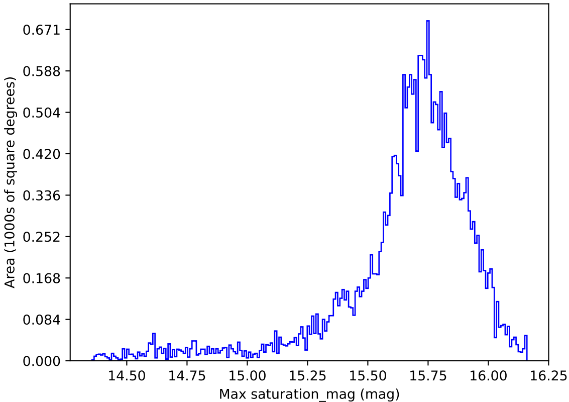
weather_cloudso4v3.4_10yrs All sky r band: Max saturation_mag
