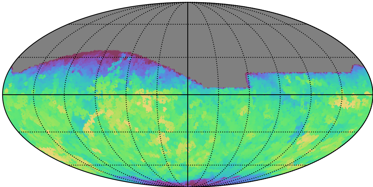
weather_cloudso4v3.4_10yrs All sky i band: Max saturation_mag
