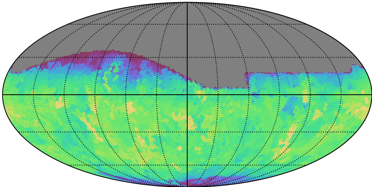
weather_cloudso4v3.4_10yrs All sky g band: Max saturation_mag
