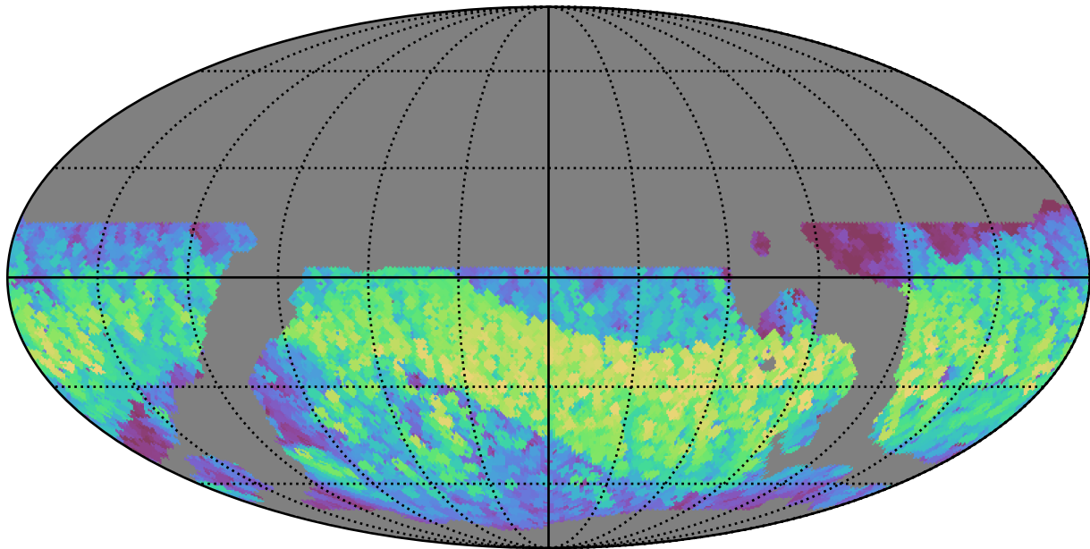
weather_cloudso4v3.4_10yrs WFD i band: Max normairmass
