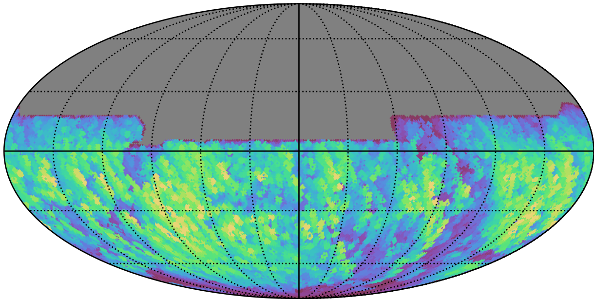
weather_cloudso4v3.4_10yrs All sky y band: Max normairmass
