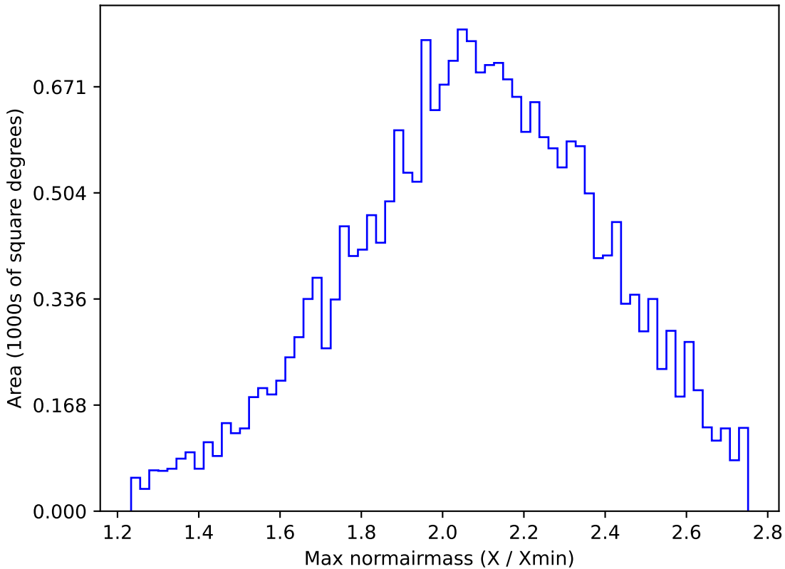
weather_cloudso4v3.4_10yrs All sky y band: Max normairmass
