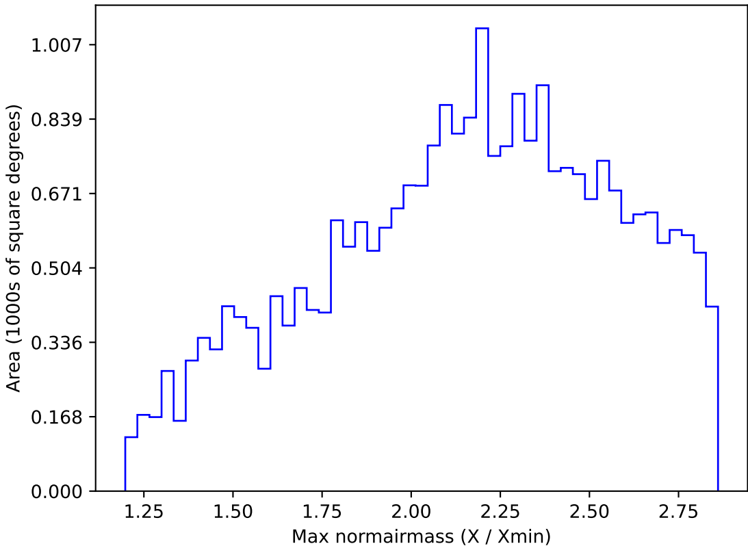
weather_cloudso4v3.4_10yrs All sky i band: Max normairmass
