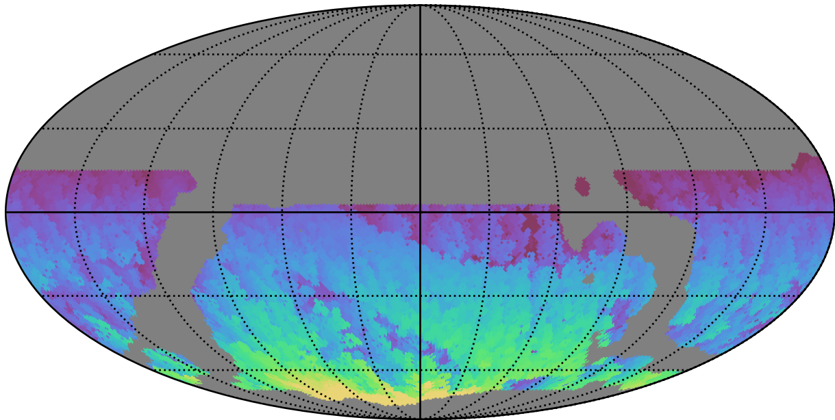
weather_cloudso4v3.4_10yrs WFD z band: Max HA
