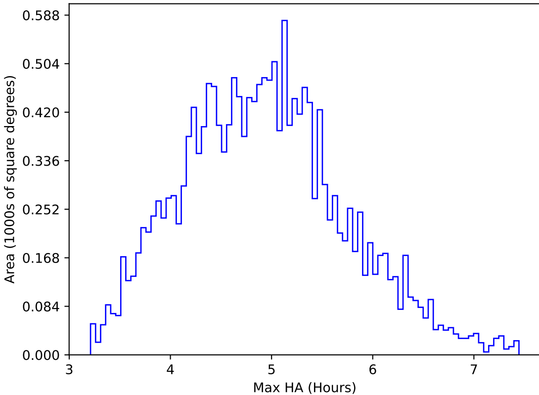
weather_cloudso4v3.4_10yrs WFD z band: Max HA
