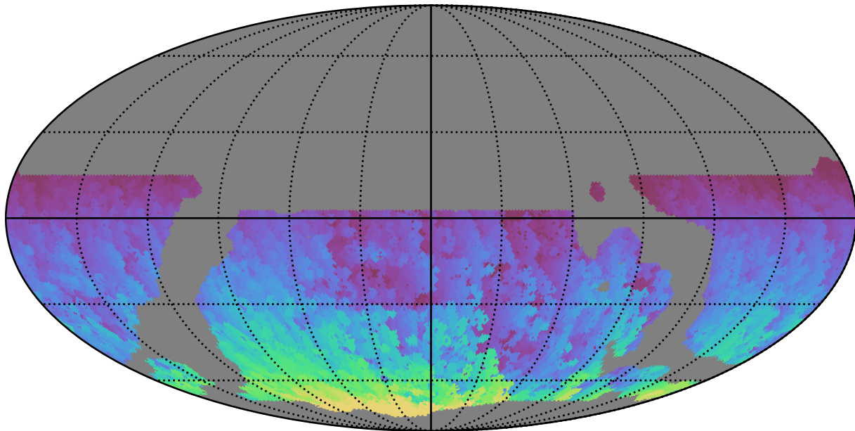
weather_cloudso4v3.4_10yrs WFD y band: Max HA
