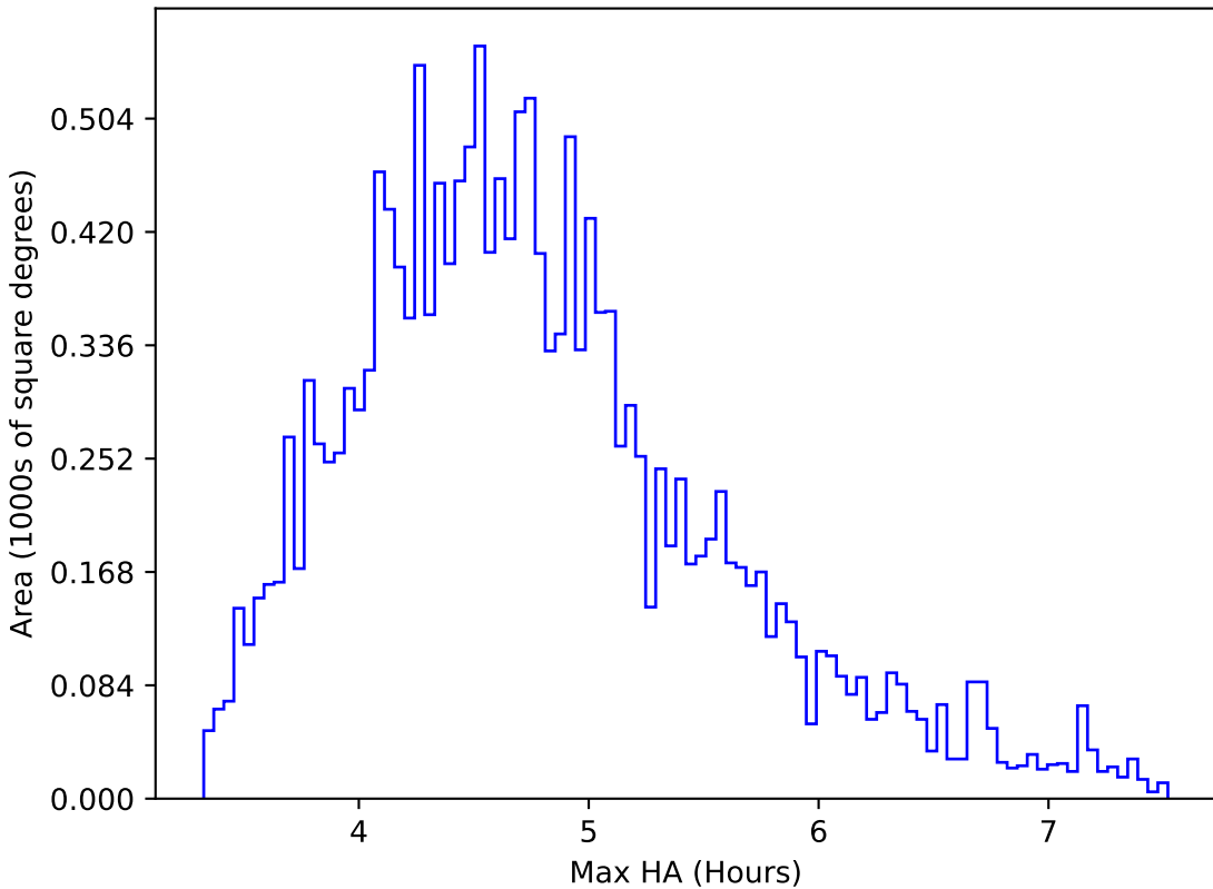
weather_cloudso4v3.4_10yrs WFD y band: Max HA
