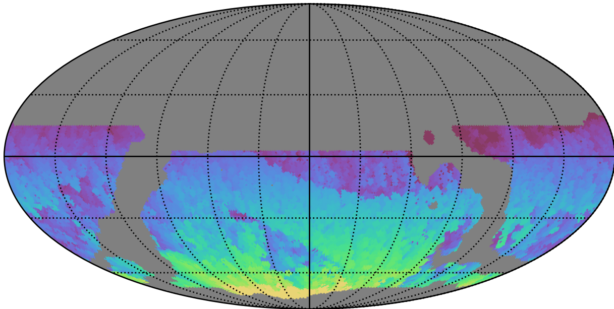
weather_cloudso4v3.4_10yrs WFD i band: Max HA
