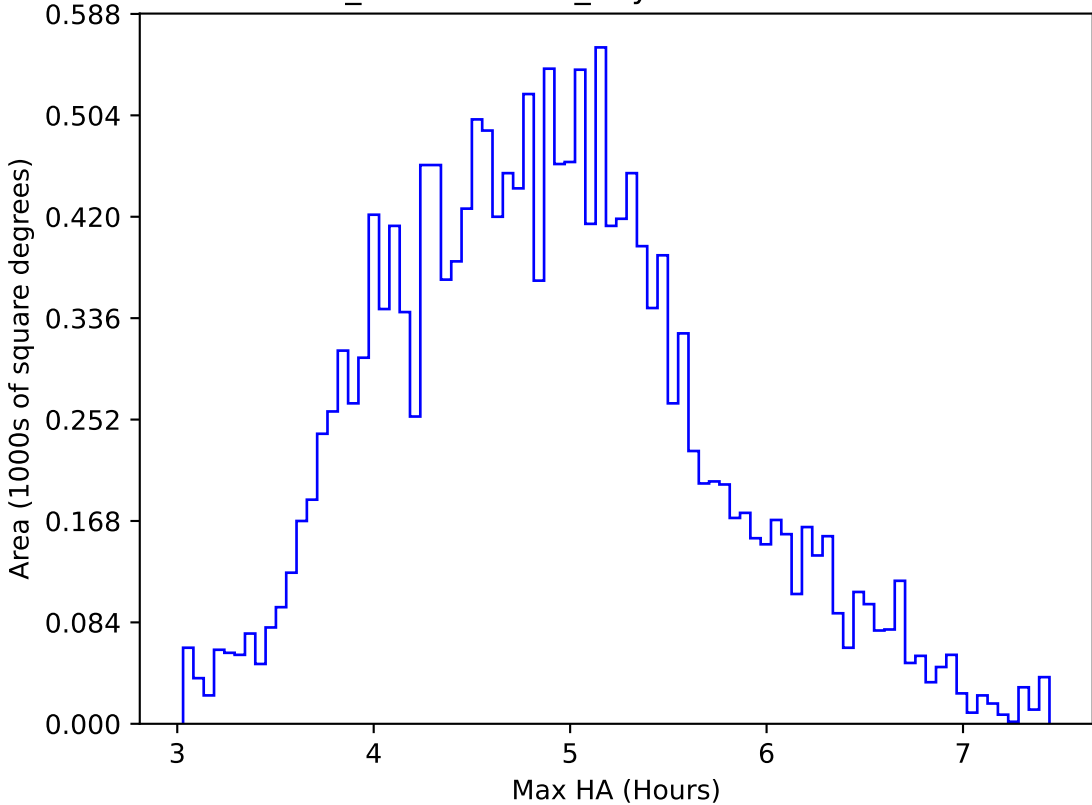
weather_cloudso4v3.4_10yrs WFD i band: Max HA
