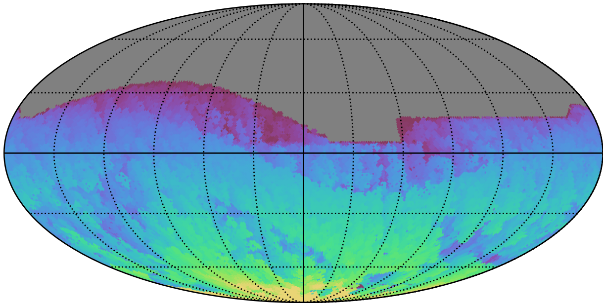
weather_cloudso4v3.4_10yrs All sky z band: Max HA
