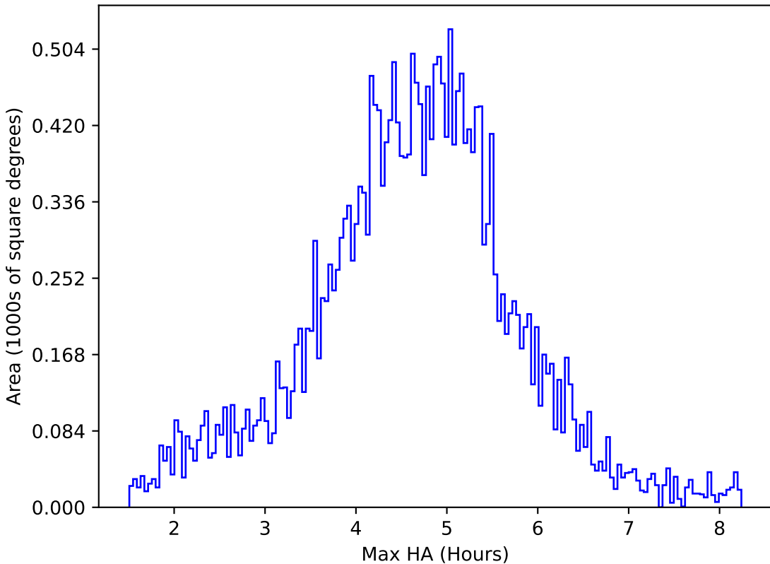
weather_cloudso4v3.4_10yrs All sky z band: Max HA
