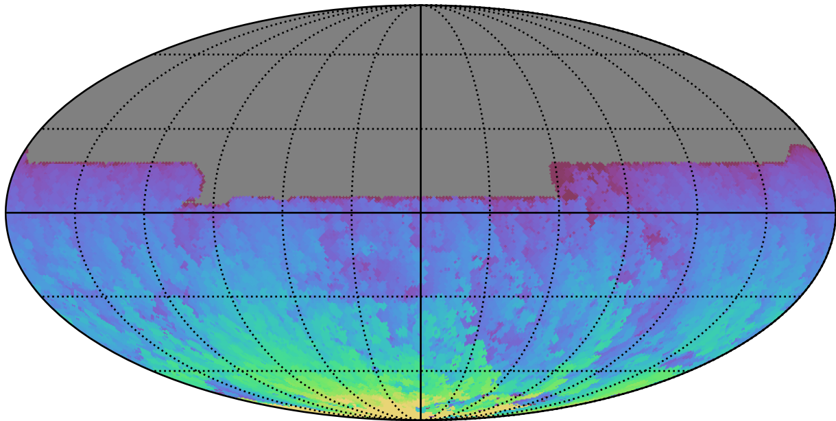
weather_cloudso4v3.4_10yrs All sky y band: Max HA
