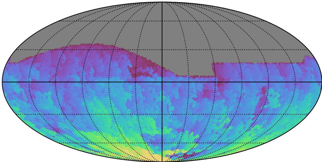
weather_cloudso4v3.4_10yrs All sky g band: Max HA
