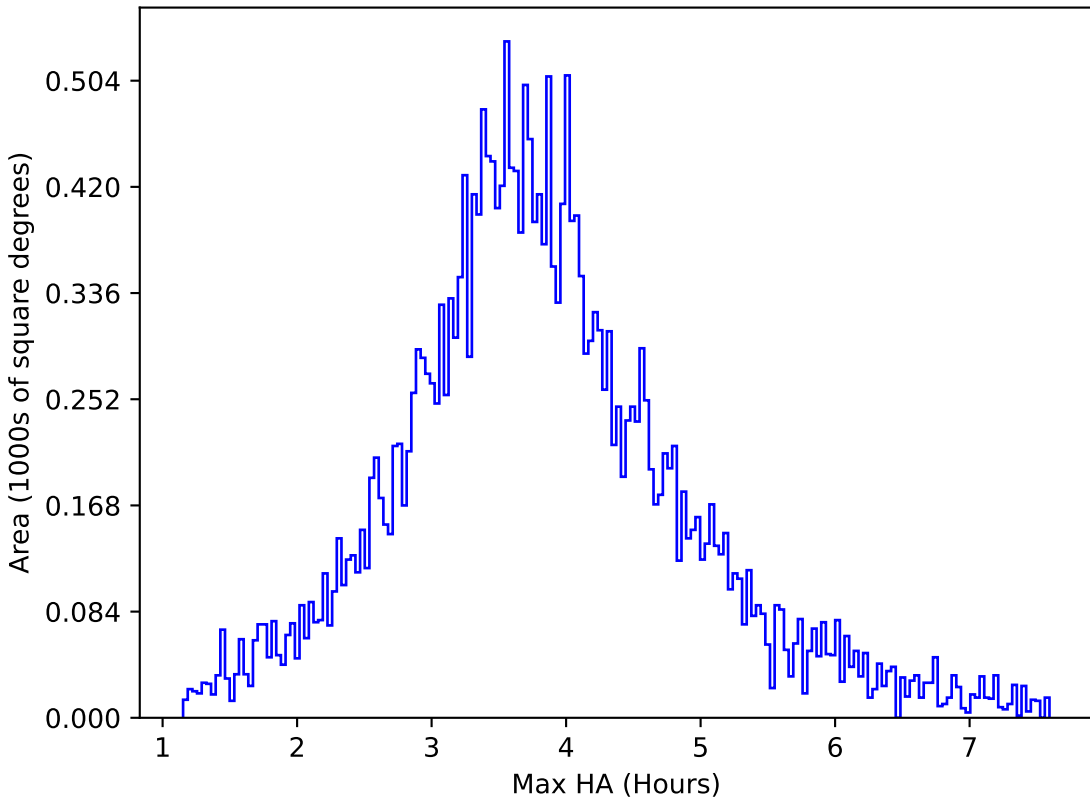
weather_cloudso4v3.4_10yrs All sky g band: Max HA
