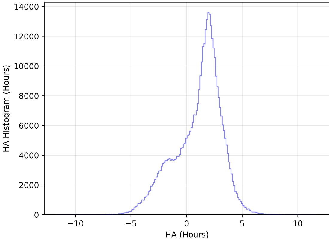
weather_cloudso4v3.4_10yrs WFD y band: HA Histogram
