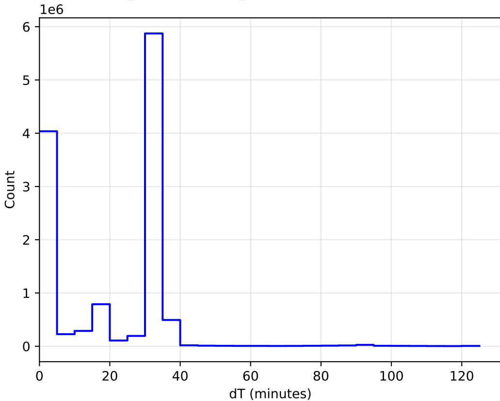
weather_cloudso4v3.4_10yrs WFD: DeltaT Histogram
