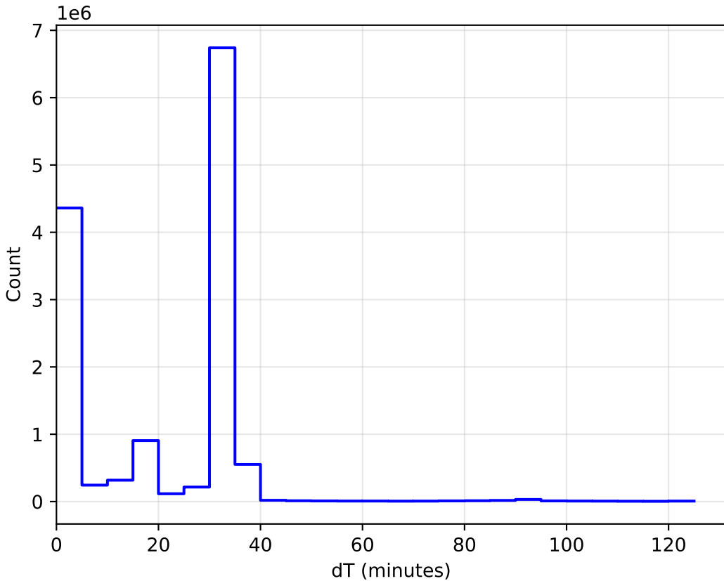
weather_cloudso4v3.4_10yrs All sky: DeltaT Histogram
