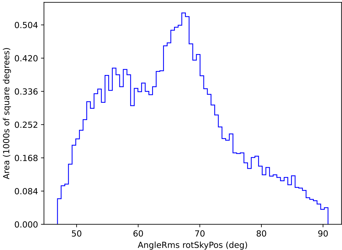
weather_cloudso4v3.4_10yrs WFD i band: AngleRms rotSkyPos
