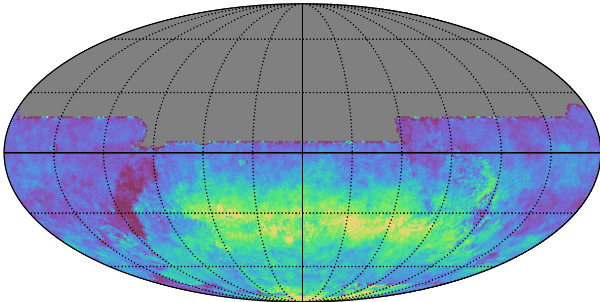
weather_cloudso4v3.4_10yrs All sky y band: AngleRms rotSkyPos
