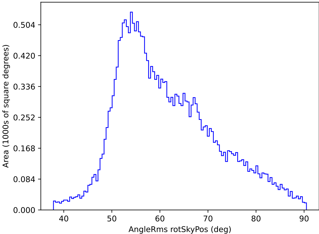
weather_cloudso4v3.4_10yrs All sky y band: AngleRms rotSkyPos
