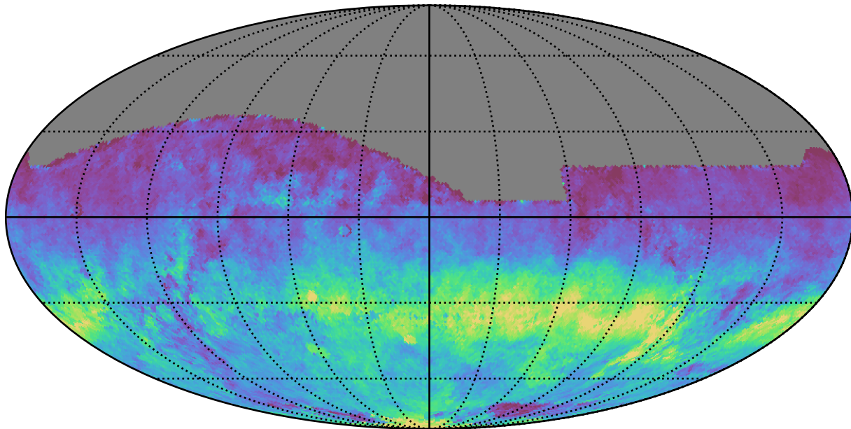
weather_cloudso4v3.4_10yrs All sky i band: AngleRms rotSkyPos
