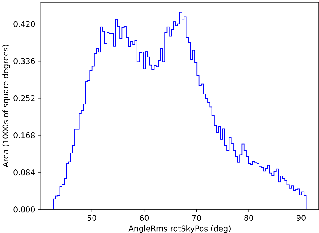
weather_cloudso4v3.4_10yrs All sky i band: AngleRms rotSkyPos
