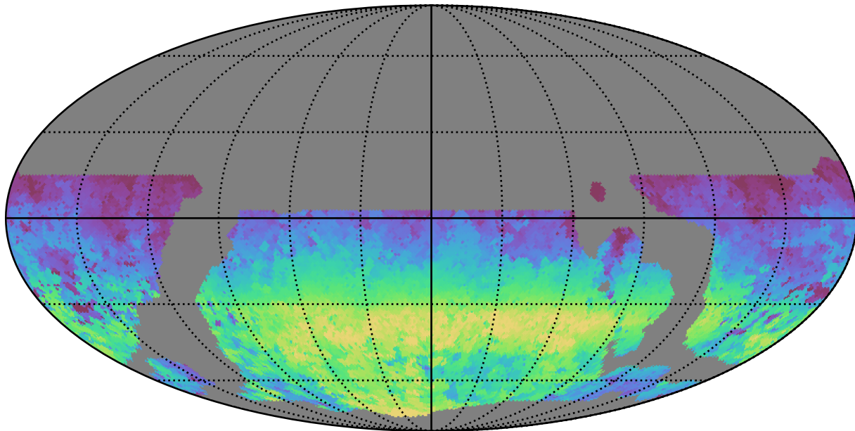
weather_cloudso4v3.4_10yrs WFD y band: AngleRange rotSkyPos
