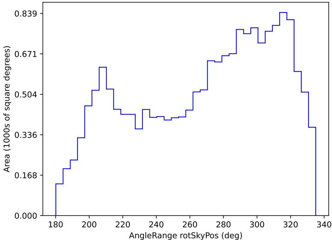
weather_cloudso4v3.4_10yrs WFD g band: AngleRange rotSkyPos
