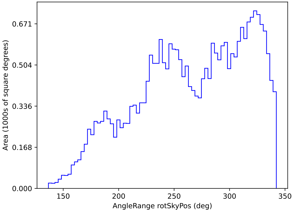
weather_cloudso4v3.4_10yrs All sky z band: AngleRange rotSkyPos
