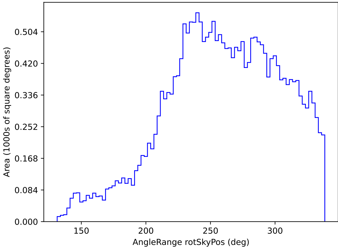
weather_cloudso4v3.4_10yrs All sky y band: AngleRange rotSkyPos
