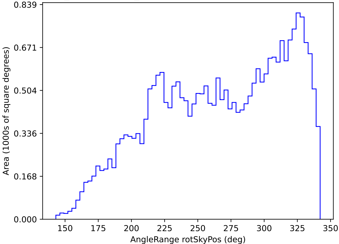
weather_cloudso4v3.4_10yrs All sky r band: AngleRange rotSkyPos
