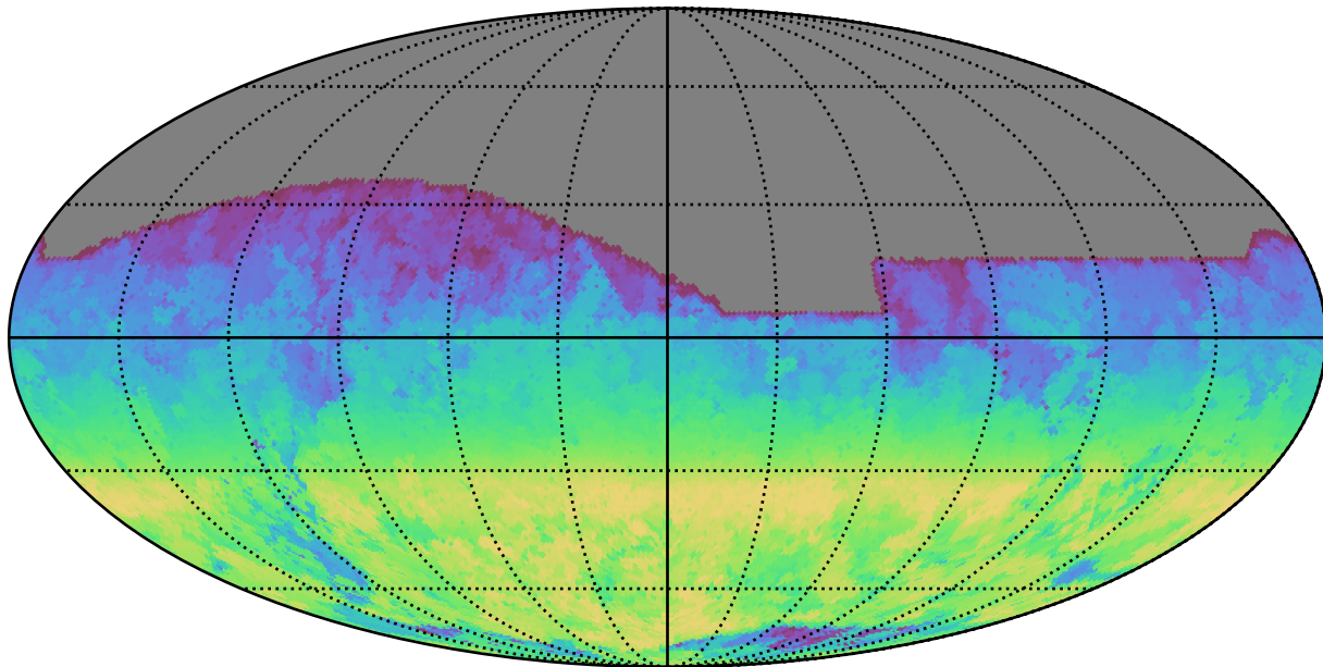
weather_cloudso4v3.4_10yrs All sky i band: AngleRange rotSkyPos
